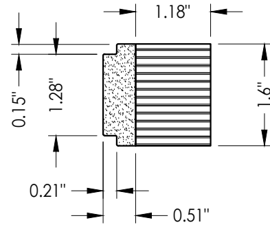
32 HINGE STILE
