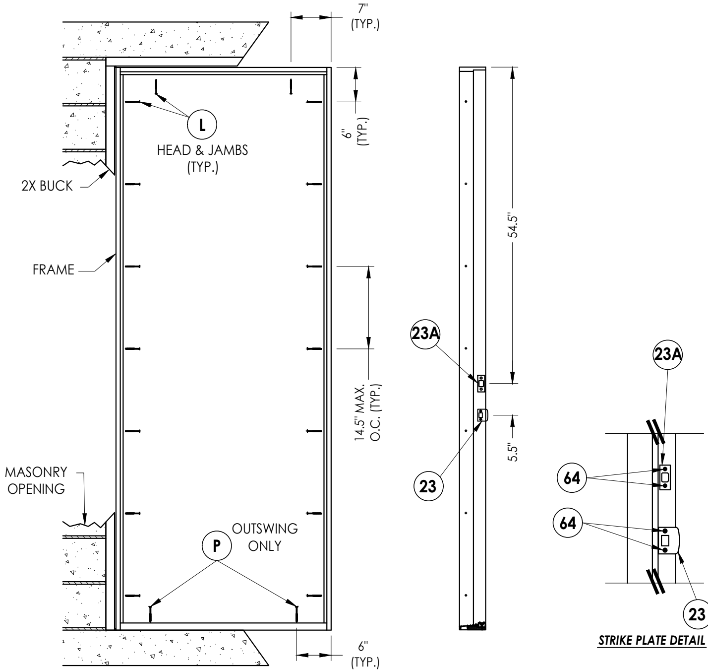
STRIKE JAMB
